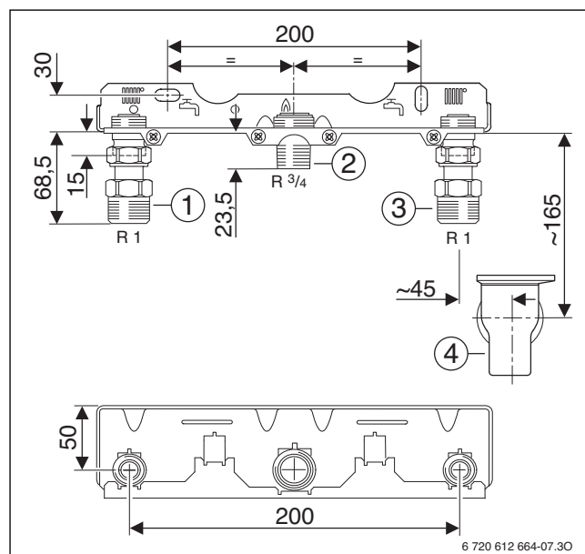
Σχ. 16 Παράδειγμα: Πλάκα σύνδεσης συναρμολόγησης αρ. 759 σε λέβητες ZBR
