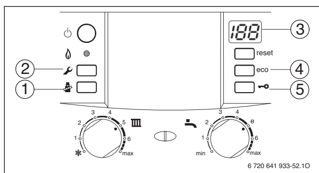
Σχ. 52 Επισκόπηση των στοιχείων χειρισμού
