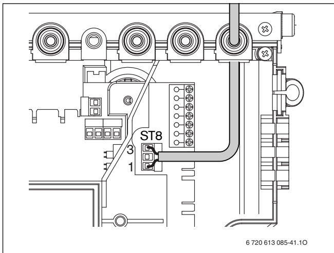
Σχ. 32 Σύνδεση θερμοστάτη μπόιλερ
