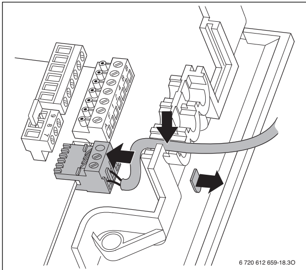
Σχ. 31 Σύνδεση αισθητήρα θερμοκρασίας μπόιλερ (NTC)
