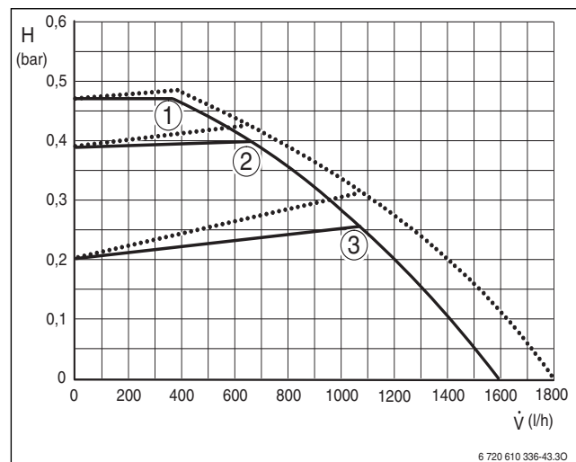
Σχ. 54 Συνεχής πίεση
