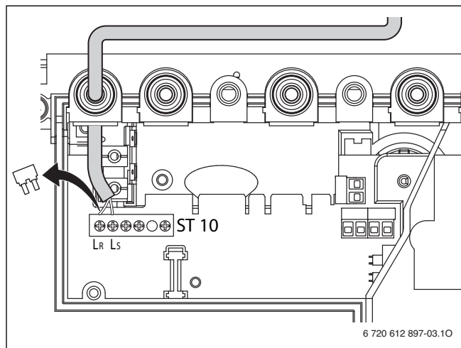
Σχ. 29 Σύνδεση (230 V AC, αφαίρεση γέφυρας μεταξύ L S και L R )
