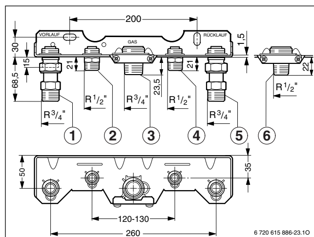
Σχ. 15 Πλάκα σύνδεσης συναρμολόγησης αρ. 258 σε λέβητες Z.BR
