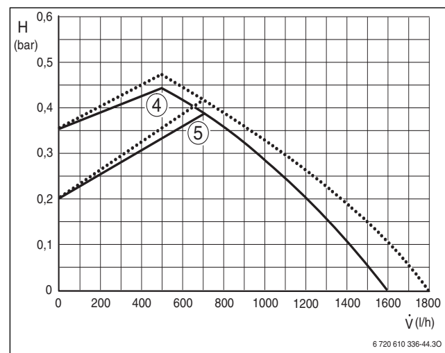
Σχ. 55 Αναλογική πίεση
