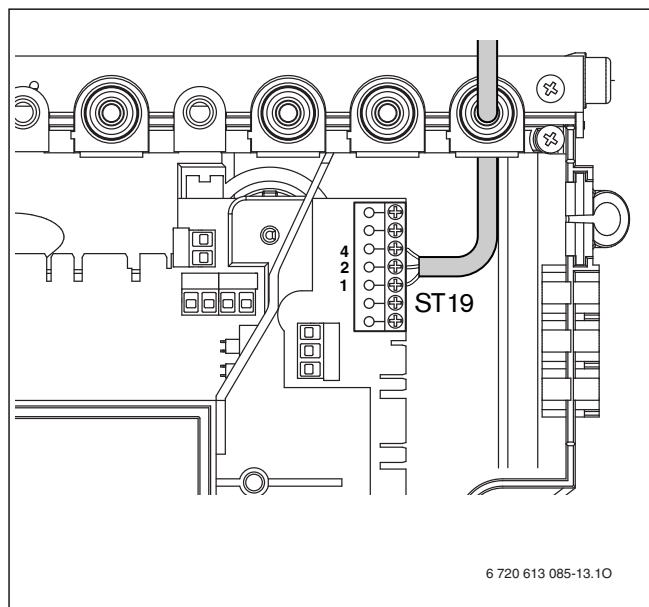
Σχ. 30 Σύνδεση συστήματος ελέγχου 24 V
