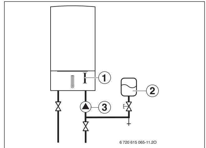
Σχ. 10 Παράδειγμα εγκατάστασης Υδραυλικό σύστημα
