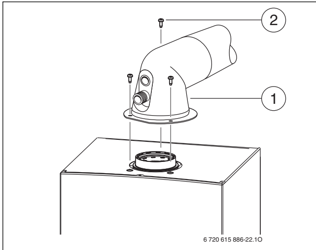
Σχ. 20 Στερέωση εξαρτήματος καυσαερίων
