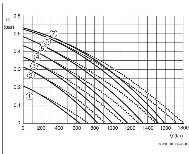
Σχ. 56 Χαρακτηριστικές καμπύλες κυκλοφορητή
